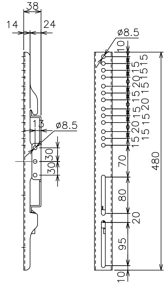
アタッチメント穴位置図
