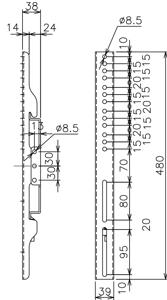
アタッチメント穴位置図
