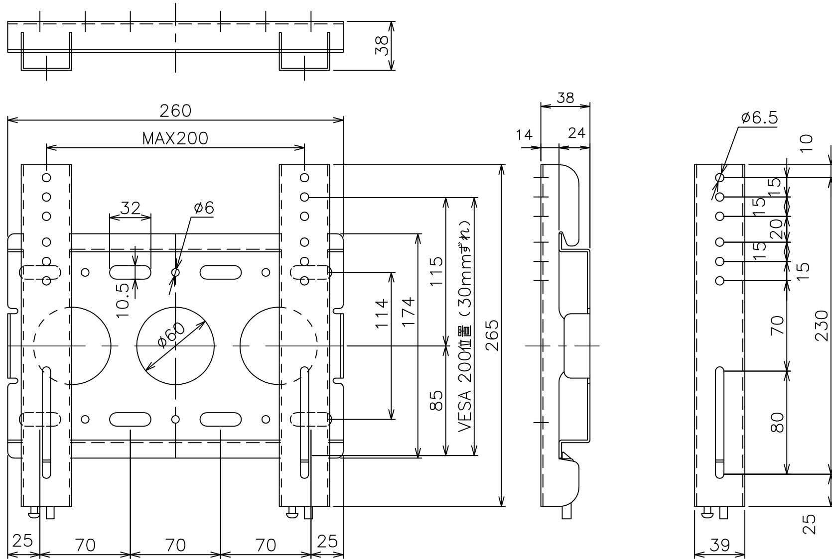
アタッチメント穴位置図
