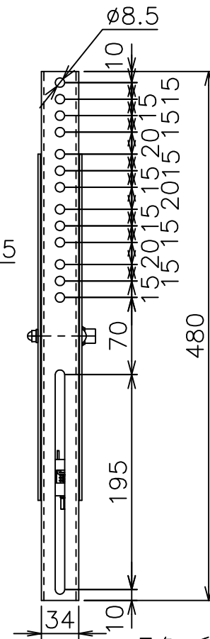
アタッチメント穴位置図
